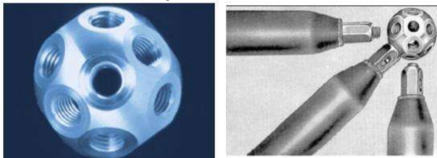
Figura 4: Sistema Mero.
