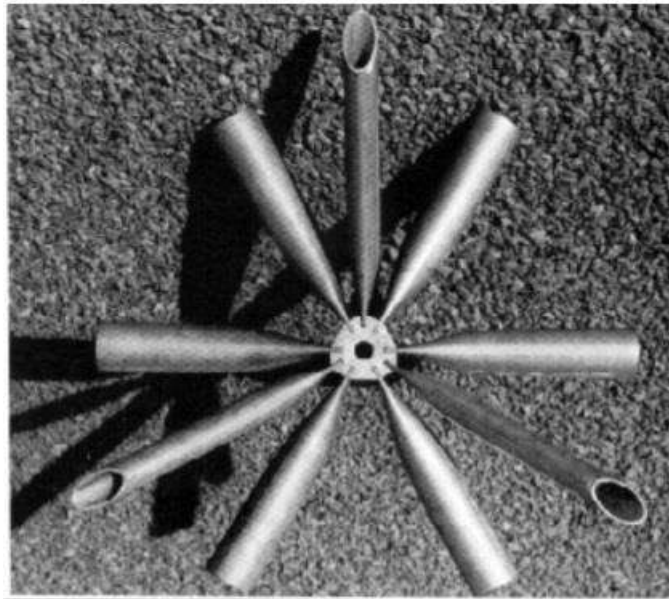
Figura 6: Sistema Triodetic.
